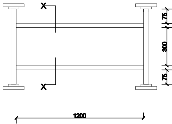
PLAN 1:25
