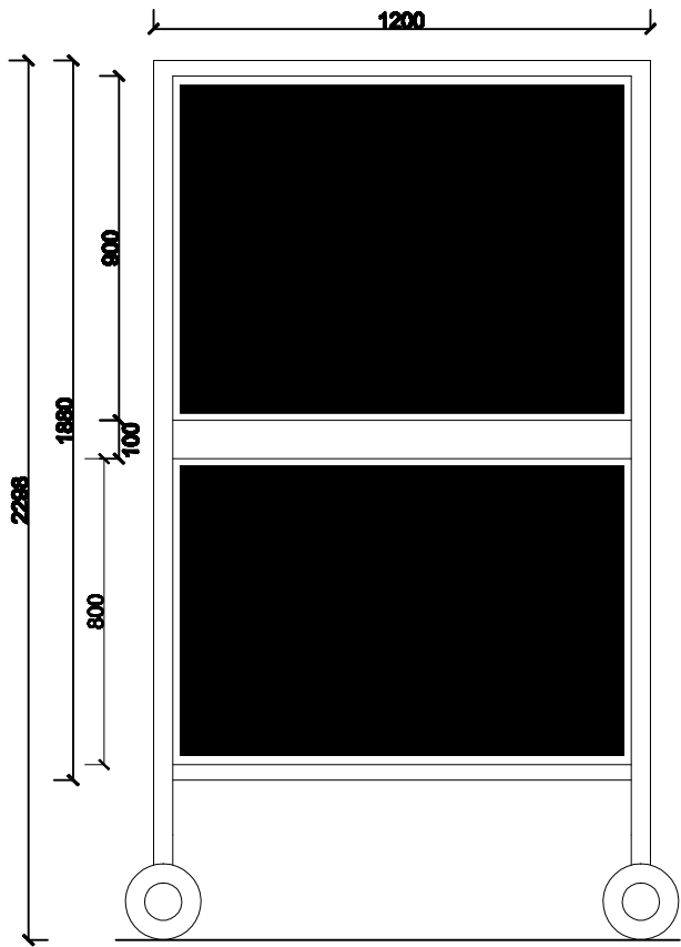
ELEVATION 1:25
